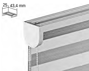
Plafondmontage met montageclip
