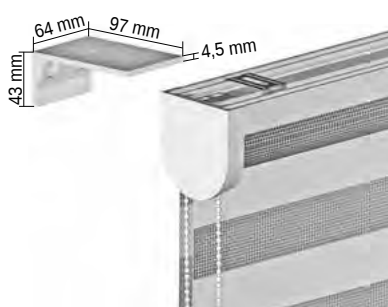
Wandmontage met wandsteun
