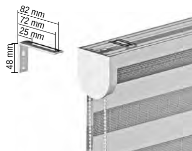
Wandmontage met hoeksteun.
