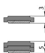
etc. Profilé de compensation de distance 21 20 13.02
