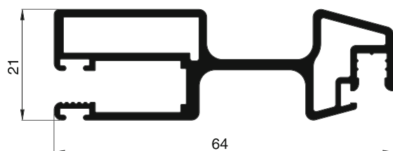
10 49 02 Profilé de vantail coulissant
