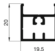
10 45 14 (uniquement disponible en G5 et S1) Coulisse droite avec canal à visser
