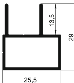
10 48 21 Rail double latéral / en haut
