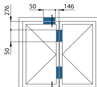
En bas avec cornière ou profilé de seuil
