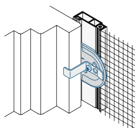
Par ex. arrêt médian SP6
