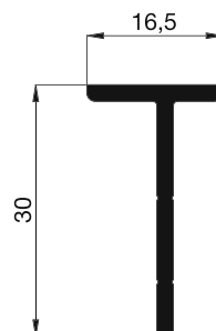
10 45 40 (uniquement disponible en G5 et S1) Profilé de montage
