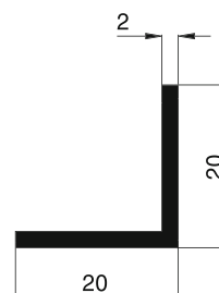
10 90 42 Cornière 20/20/2 pour recouvrement de puits de lumière
