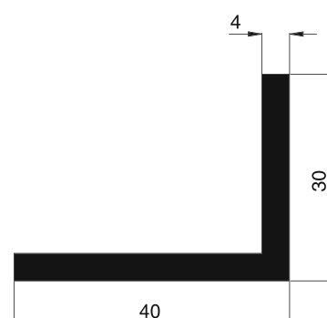
10 90 90 (uniquement disponible brut) Cornière 40/30/4
