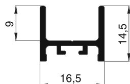
10 48 20 Rail double en bas
