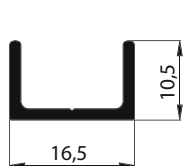
10 48 19 (uniquement disponible en E1) Rail double plat en bas
