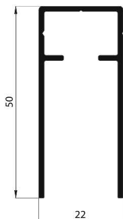
10 45 02 Profilé haut 50 mm
