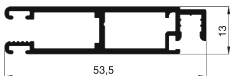
10 48 02 Profilé de vantail coulissant
