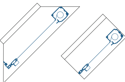
Montage sur une fenêtre à ouverture par pivot central
