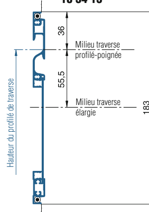
avec traverse profilé-poignée 10 34 13
