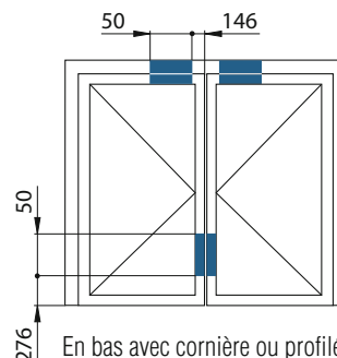
En bas avec profilé de cadre de montage
