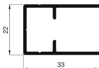
10 45 04 Profilé de cadre
