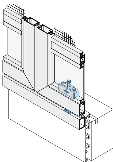
Blocage de vantail semi-fixe verrouillé (fermé)
