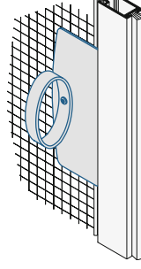
Boucle textile 13 35 57 Plaque de protection 13 35 51
