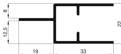
10 45 06 Profilé de cadre
