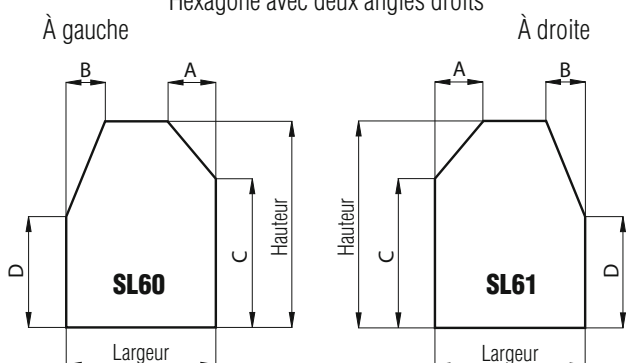
Hexagone avec deux angles droits
