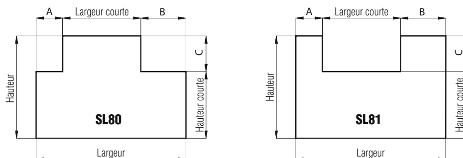
Octogone avec huit angles droits
