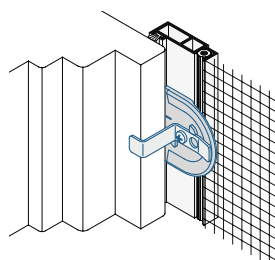
Par ex. Arrêt médian SP2
