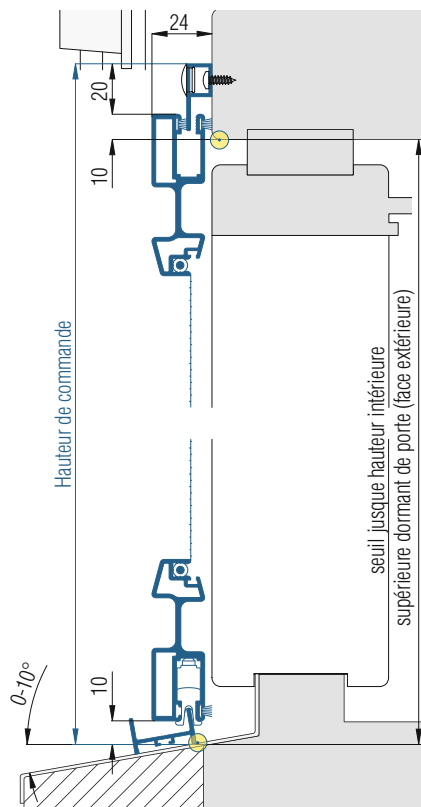
Coupe verticale, échelle 1:3
