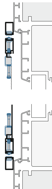
Blocage de vantail semi-fixe déverrouillé (ouvert)
