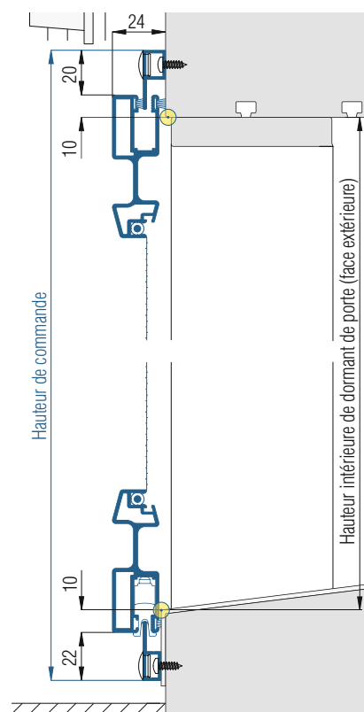
Coupe verticale, échelle 1:3
