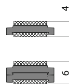
etc. Profilé de compensation de distance 21 20 13.02
