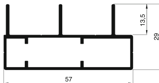
10 49 31 Rail triple latéral / en haut / en bas
