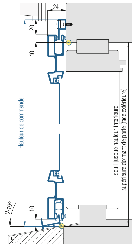
Coupe verticale, échelle 1:3
