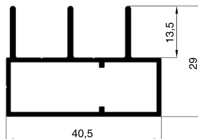
10 48 31 Rail triple latéral / en haut / en bas
