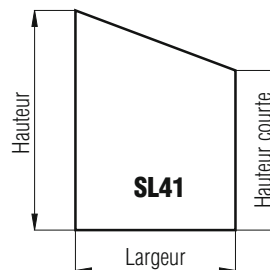
À gauche Quadrilatère avec deux angles droits À droite
