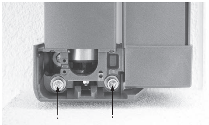
Abb. 17: Sicherungsschrauben* entfernen
