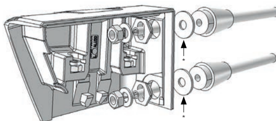
Wandkonsole auf Fischer Thermax M16 mit Unterlegscheiben* (Ø 13 mm DIN 9021) (2 Stk. pro Konsole)
