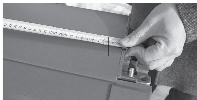
Abb. 02: Kassettenbreite messen
