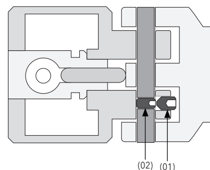
Fig. 14: support de bras articulé en coupe - vis pointeau placées l'une derrière l'autre
