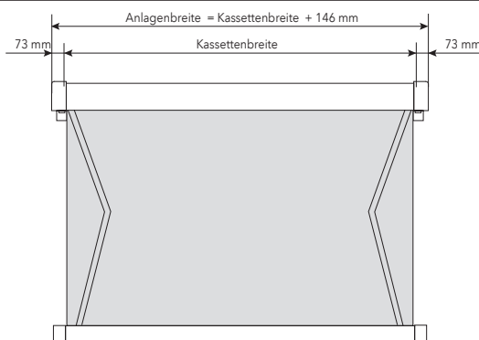
Abb. 01: Anlagenbreite
